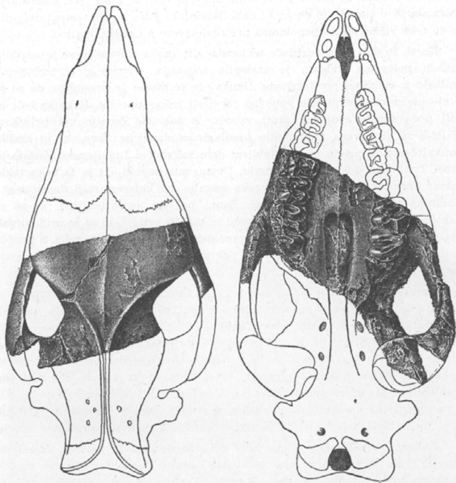
Slika 2. Rekonstruirana lobanja pritlikavega nosoroga Meninatherium teleri Abel iz oligocenskih premogovih plasti v Motniku. Našli so samo srednji, temneje risan del lobanje. Pogled od zgornje in od spodnje strani. Po Abelu.
