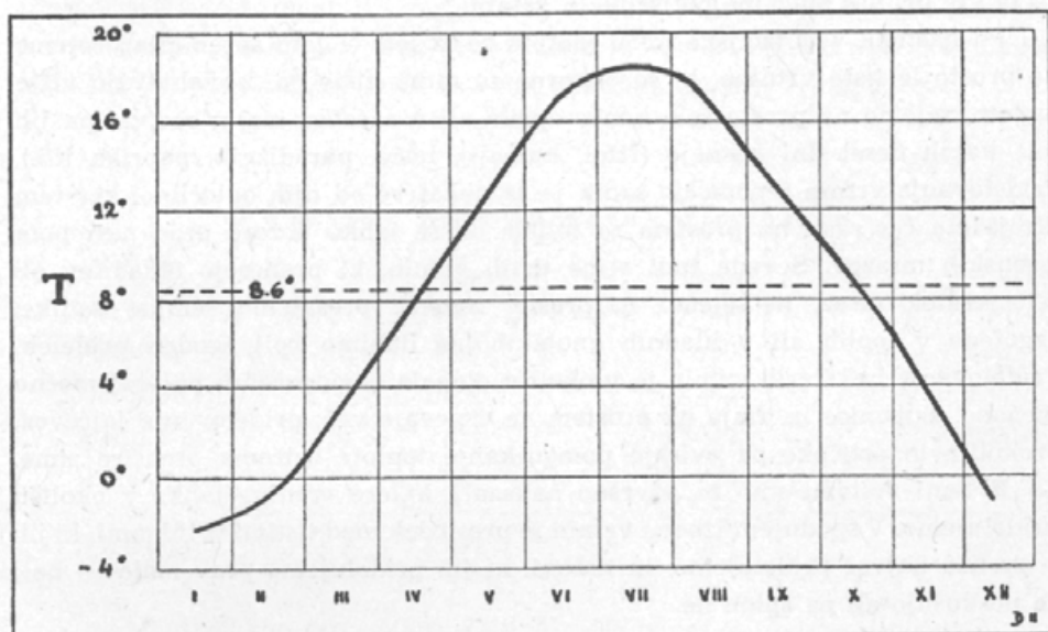
Diagram D II: Temperaturna krivulja, Kamnik 1925—1940
