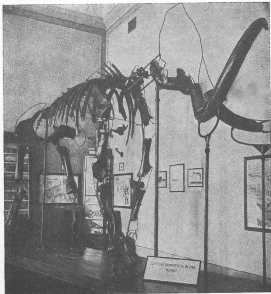
Slika 6. Okostje mamuta [ Mammonteus primigenius (Blumenb.)] izkopano pri Nevljah. Iz würmske dobe. Po Kosu.
