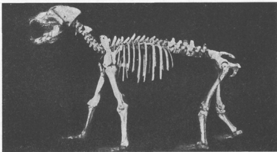
Slika 7. Okostje jamskega medveda ( Ursus spelaeus Rosenm. et Heinroth) iz Mokriške jame. Iz würmske dobe. Po Kosu.
