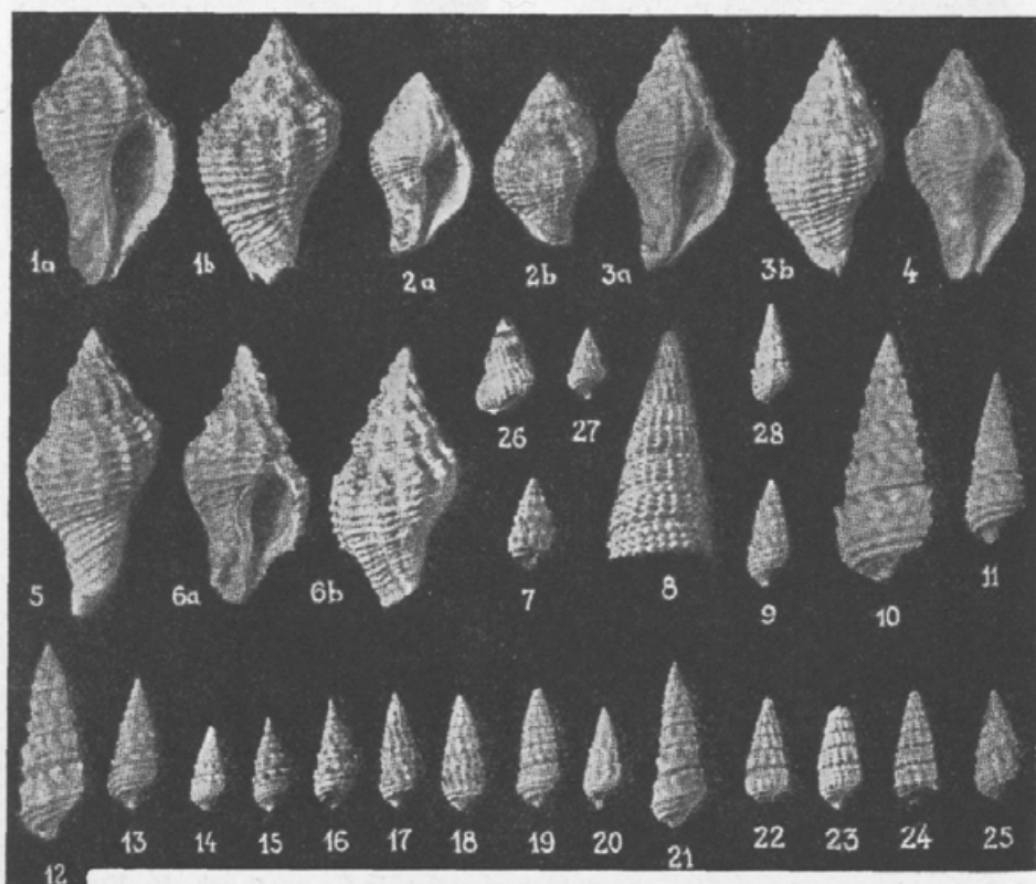
Slika 3. Polževe hišice iz miocenskih plasti v Tunjškem gričevju. 1—6 različne vrste rodu Murex , 7—25 in 27—28 različne vrste rodu Cerithium , 26 Buccinum . Vse v naravni velikosti.
