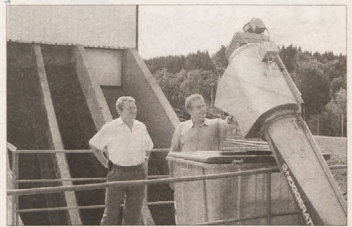
ROTOMATNI POLŽ - Vodja tehničnega sektorja Komunale Boško Vujasin in direktor Komunale Trebnje Pavel Jarc si ogledujeta eno od pridobitev prve faze prenove ČN v Trebnjem - rotomatni polž za odstranjevanje trdih delcev iz odpadka. (Foto: J. Ž.)
