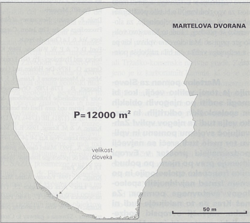
Največji prečni prerez Martelove dvorane z izmerjeno največjo višino stropa 146 metrov
