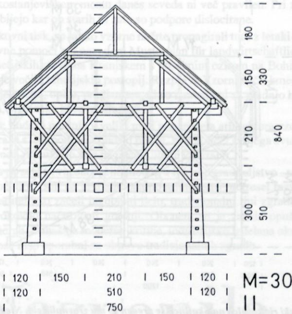
Slika 5. Naris Sotlerjevega "toplerja" na Škofljici, izdelanega v metrskih merah. Modul kompozicije je "metrski čevlj", dolžine 30 cm.
