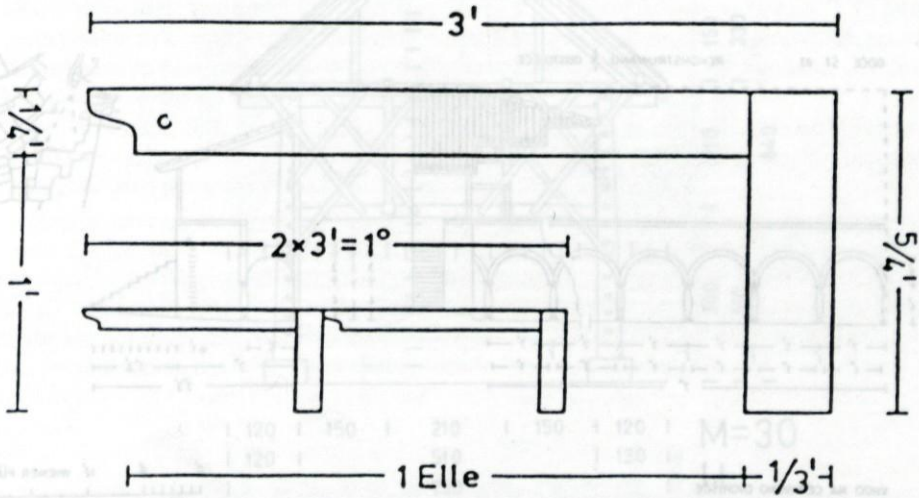
Slika 3. Tesarski "vinkl", rekonstruiran po pripovedovanju prof. Kobeta. Podobno, vendar manjše merilo v obliki črke L so imeli mizarji.
