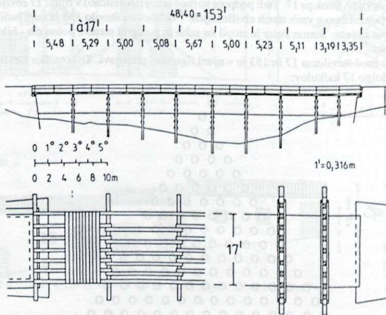
Slika 7. Leseni most čez Krko pri Kostanjevici je dolg 153 čevljev, širok pa 17. Razmak med podporniki je (teoretično) tudi po 17 čevljev. Oblikovano število 153 simbolizira ribiško mrežo.
