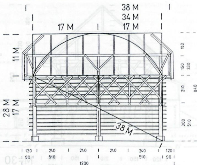
Slika 6. Stranski ris kozolca na Škofljici, še preden so mu zravnali čelo. Njegove mere, ki so zmnožek Fibonaccijevih števil z modulom, so v proporciji zlatega reza.
