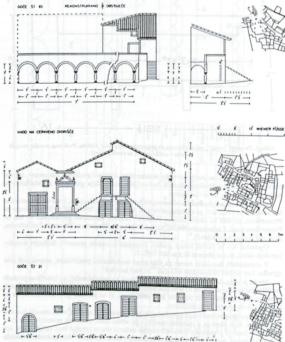
Slika 4. Hiše v Gočah so zasnovane v dunajskih merah. Kolonada v zgornji vrsti je v ritmu 7 čevljev, širina hiš v drugi vrsti je 3 klastre in pol oziroma 6 klastre. Seveda so tudi višine zgradb v dunajskih merah, prav tako pa tudi okna, vrata, stopnišča itd.
