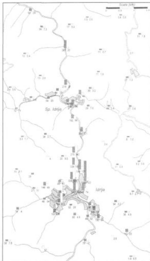
VSEBNOST ŽIVEGA SREBRA (MG/KG) V PODSTREŠNEM PRAHU (SIVO OZNAČENA) IN V ZEMLJI V OBMOKJU IDRJE GOSAR IN SOD., 2001
