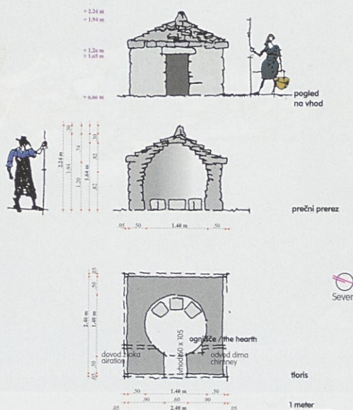
Slika 5: Osnovni načrt z vsemi potrebnimi tehničnimi podatki. Vnešene so razsežnosti, višinske kote in nujni opisi detajlov. Analize (predvsem proporcijška) so poseben projekt pri zasnovi načrtovanja.
