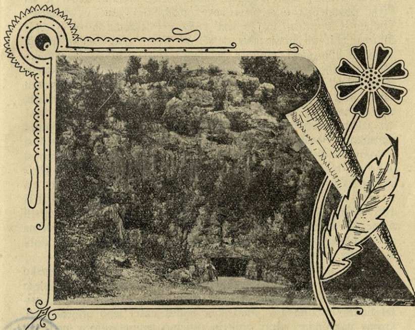
Uhod v Otoško jamo.
