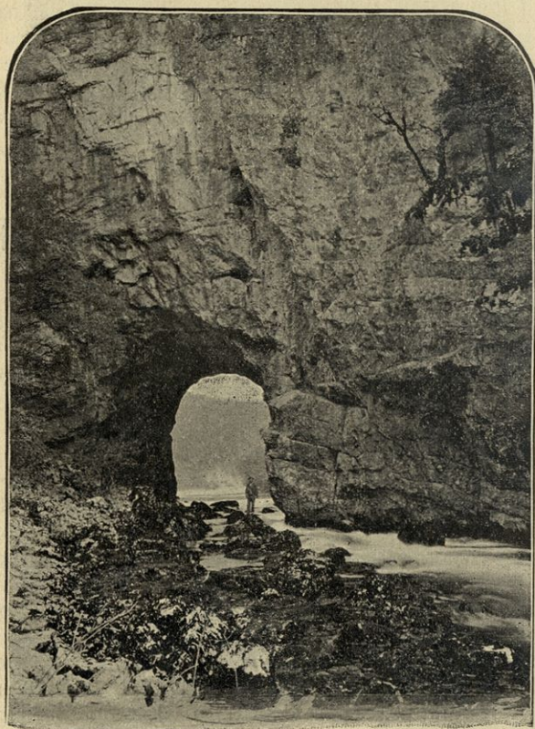
Škocijanski veliki naravni most od južne strani.
