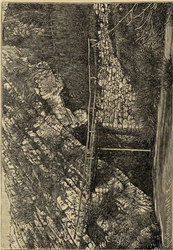
Odtok Pivke v postojnsko jamo.
