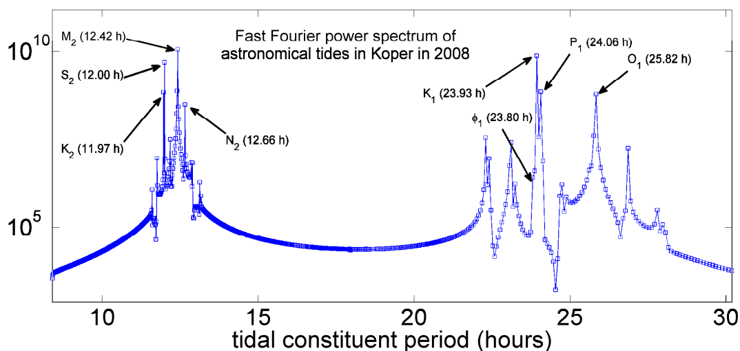
Slika 2: FFT spekter višin morja na mareografski postaji Koper za leto 2008. Označene so periode osnovnih dnevnih in poldnevni plimnih komponent.
