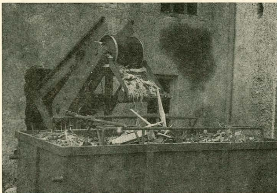
Mehaniziran transport lubja in lesnih ostankov od obeh polnojarmenikov iz žagalnice v Mislinji
