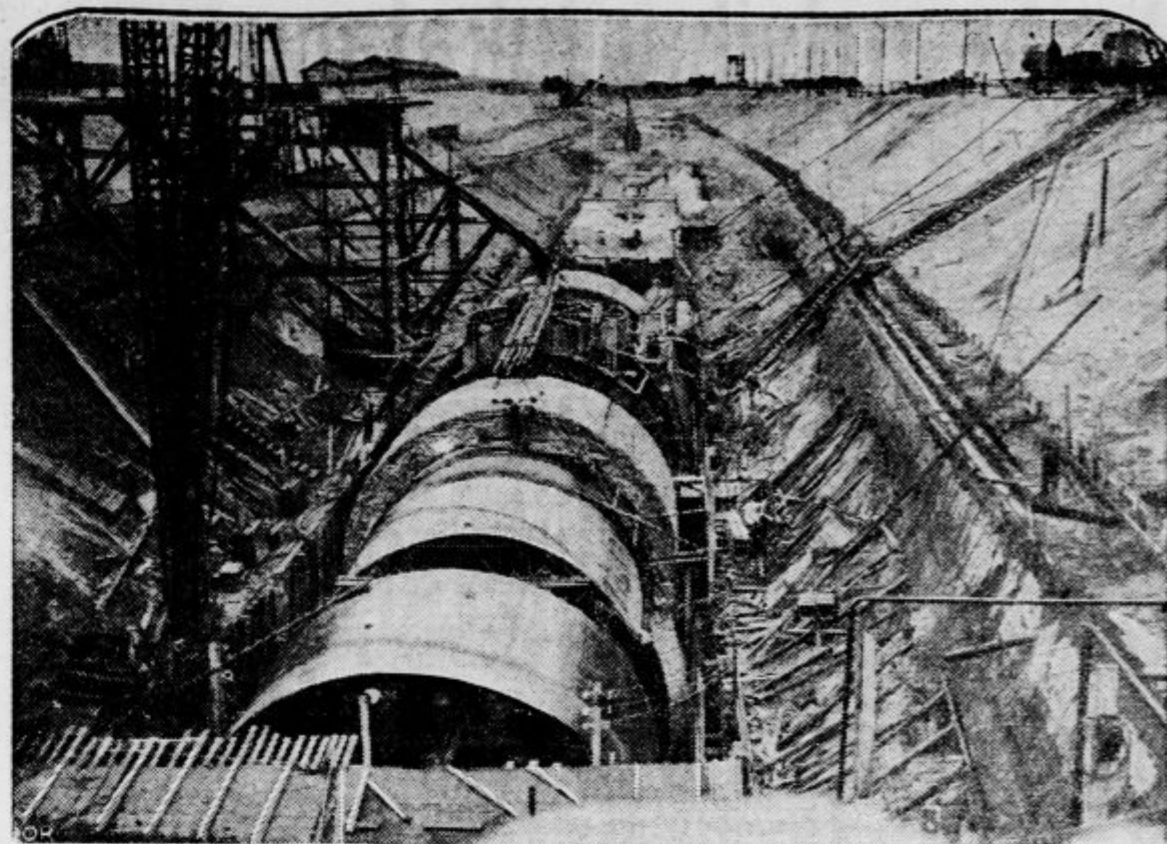
Predor pod reko Escaut (Skajda) bo služil za promet pešcev in vozil. Slika kaže enega izmed vhodov v predor. Vidijo se ogromni betonski obodi, ki bodo tvorili stene predora.
