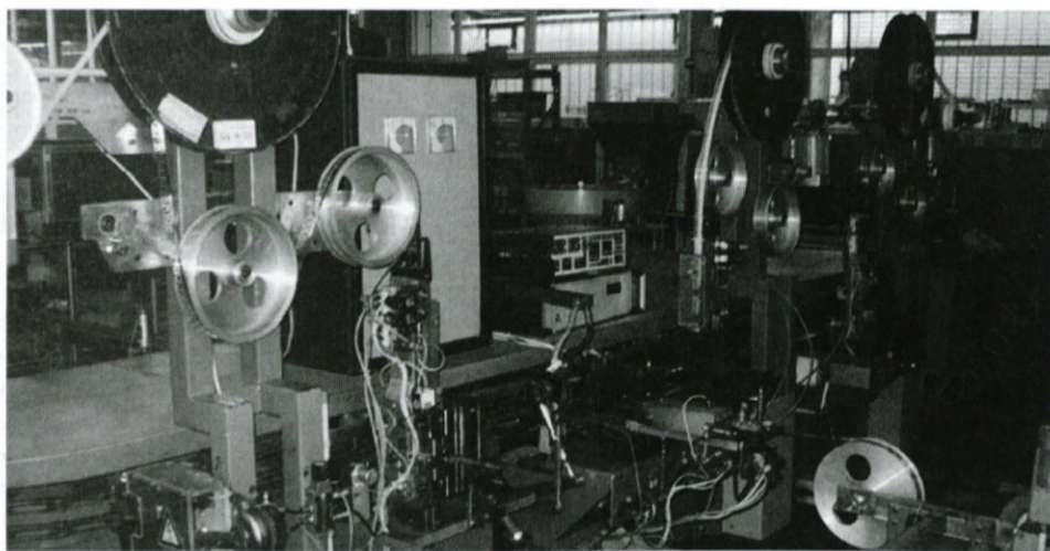
Detajl iz prve avtomatizirane linije v ISE. (Foto: Ivan Grandovec, maj 2005).
