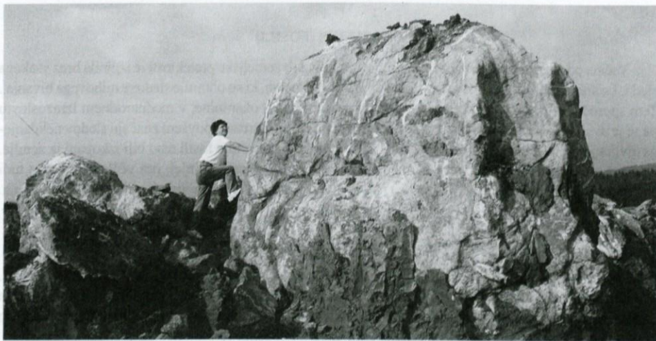
Ko hodimo po zemlji, se večinoma ne zavedamo, da je pod nami orjaško skalovje - pravi planinski svet. Pogled na odkrito površino ob gradnji avtomobilske ceste. Vodotučine pri Ivančni Gorici, 1999.
