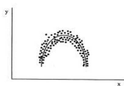
Slika 1.7: Nelinearna oblika povezanosti med spremenljivkama x in y
