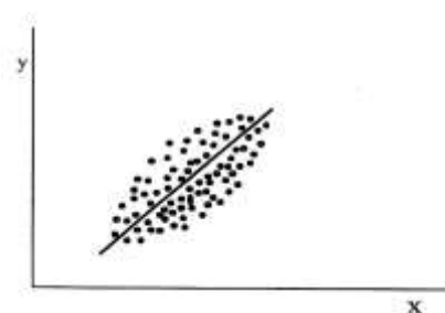
Slika 1.6: Linearna oblika povezanosti med spremenljivkama x in y
