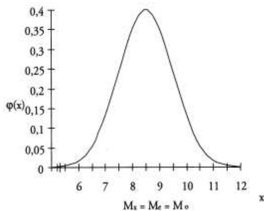
Slika 2.1: Graf normalne porazdelitve
