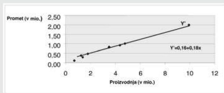
Slika 1.8: Razsevni diagram in regresijska premica za število zaposlenih v prometu in proizvodnji v nekaterih državah evropskega prostora za leto 1991
