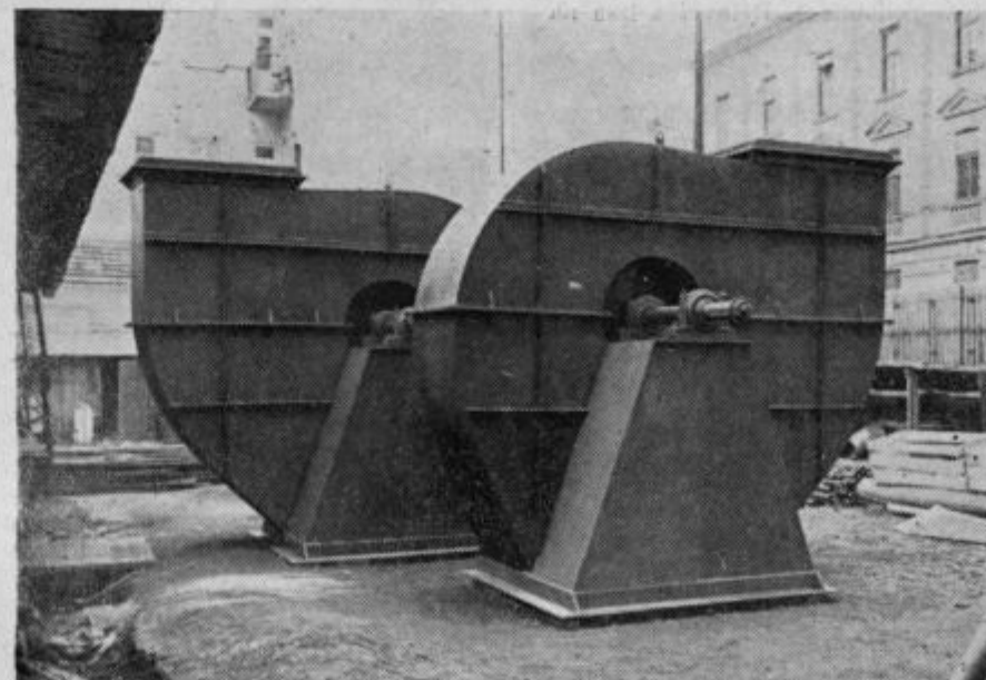
Na ta dva ventilatorja, ki so ju izdelali za rudnik Kakanj, je kolektiv še posebno ponosen. Vsak je visok 3 in pol metra, dočim je premer rotorjev 2 metra in tehta ca. 3.800 kilogramov. Pogonski elektromotor s 105 KW poganja omenjeni ventilator
