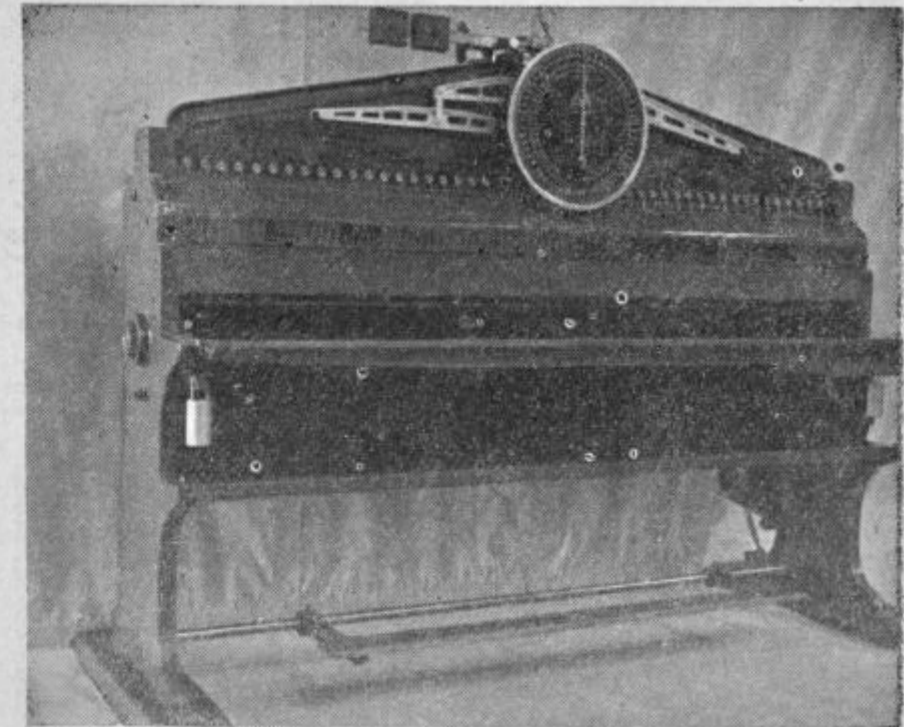
Merilni stroj za površinsko merjenje usnja »Kostroj«
