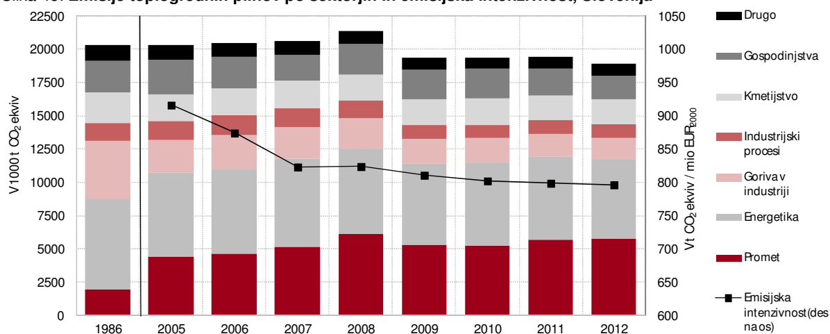
Slika 45: Emisije toplogrednih plinov po sektorjih in emisijska intenzivnost, Slovenija
