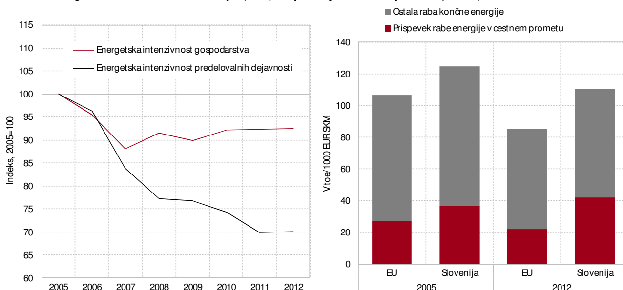
Slika 46: Energetska intenzivnost, Slovenija, (levo) ter primerjava Slovenije in EU (desno)
