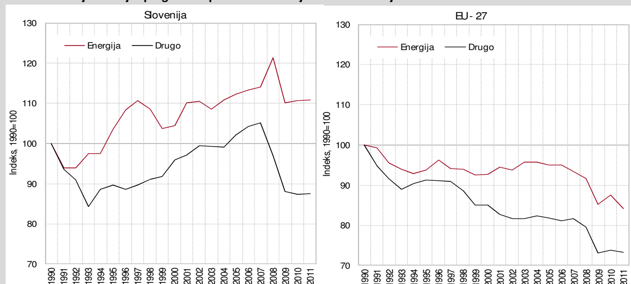
Slika 1: Gibanje emisij toplogrednih plinov v Sloveniji in EU v obdobju 1990 – 2011
