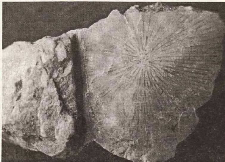
korala DIPLAREA ELEGANS , zg. jura, Otlica 3/B foto: FOTO GO
