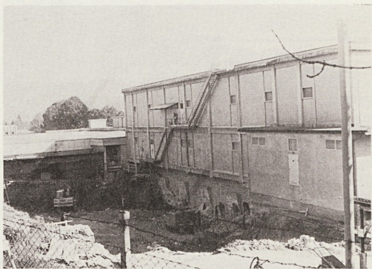
Pred letom dni smo pričeli graditi prizidek predilnice, danes pa je že pripravljen za montažo strojev. Na sliki — izkop temeljev za prizidek.
