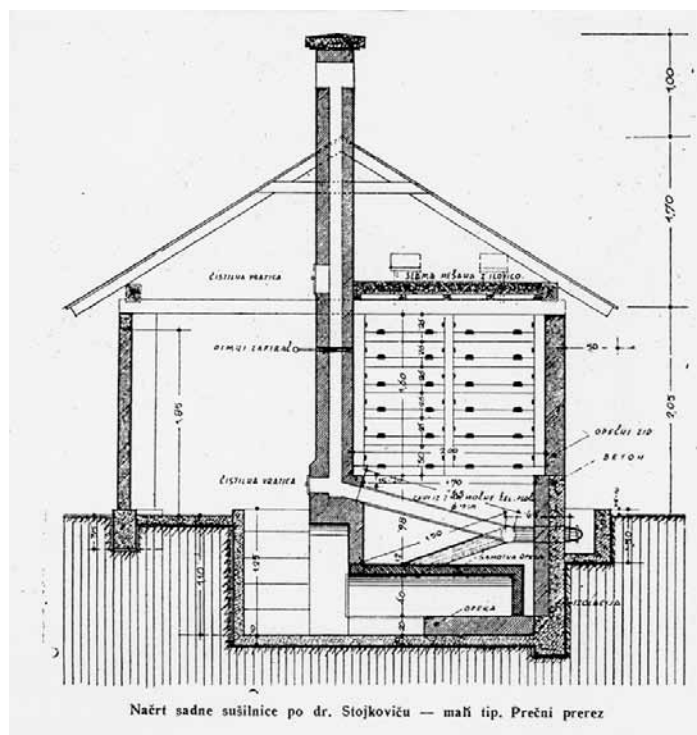
Načrt sadne sušilnice po dr. Stojkoviću, mali tip. Prečni prerez.
