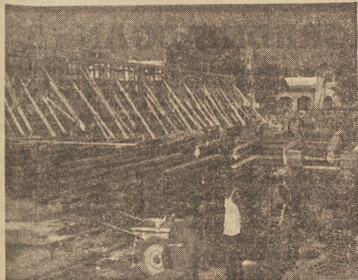
Del gradbišča nove predilnice v Ajdovščini
