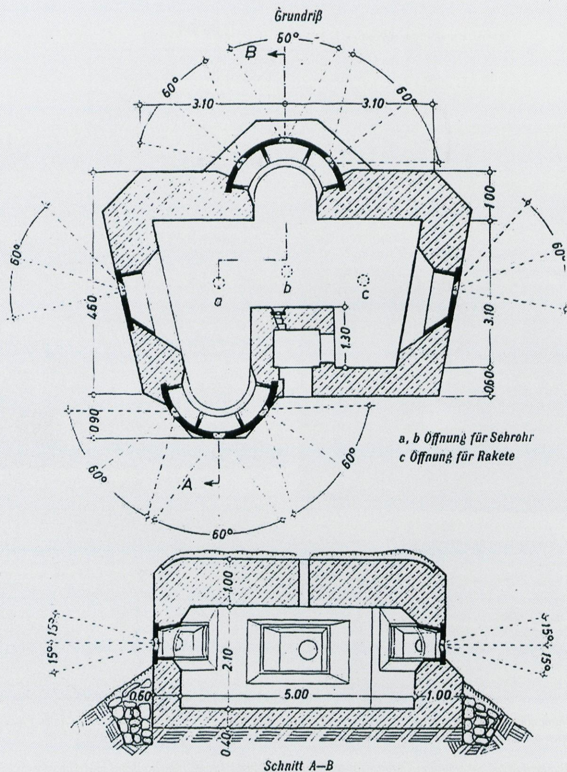
M. G.-Stand mit zwei dreifachen gebogenen und zwei einfachen Panzerscharten
