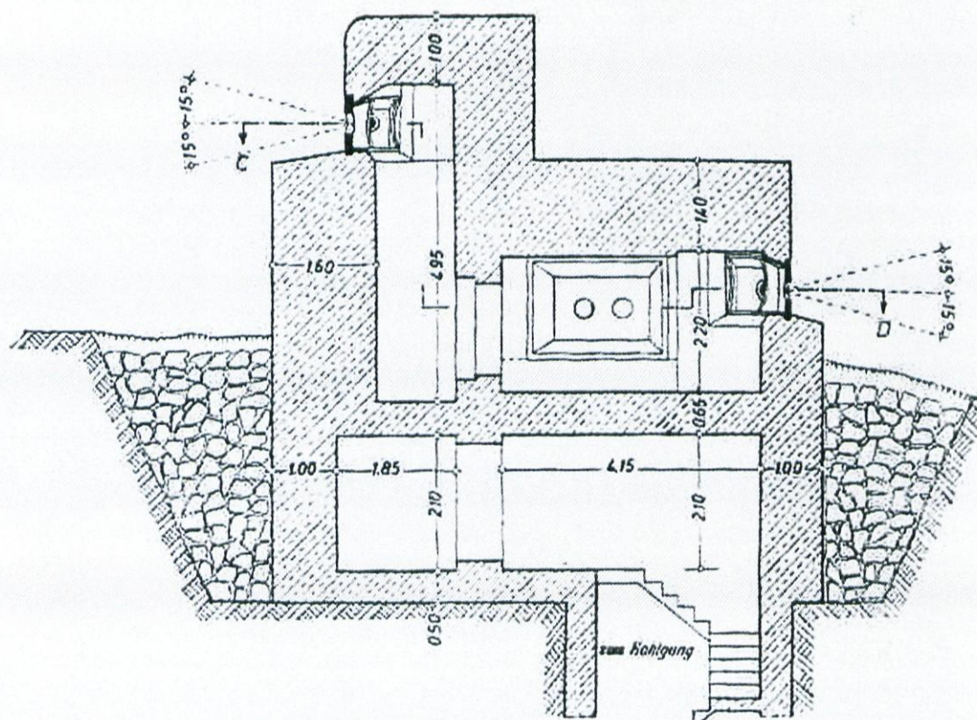
Schnitt A—B
