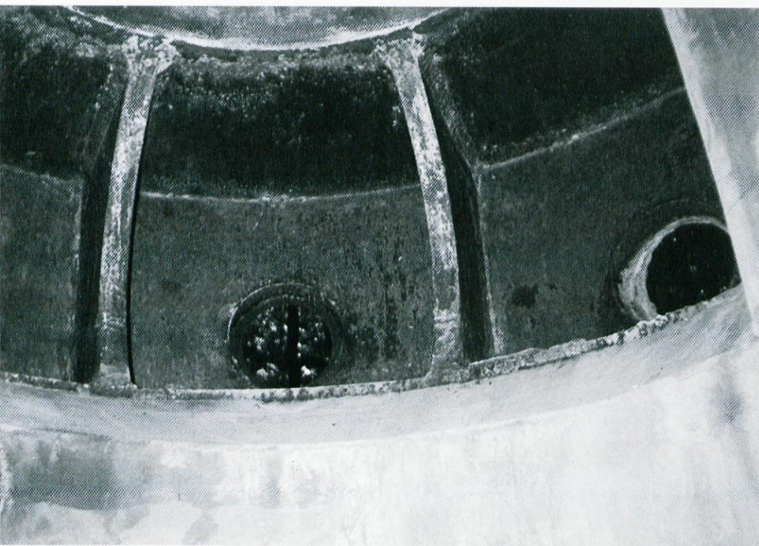
Značilna, z navpičnimi rebri okrepljena polkrožna plošča s tremi okroglimi strelskimi linami – zaščitni znak utrdb Rupnikove linije na tem sektorju
