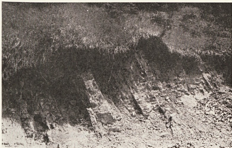
Sl. 21. Plastnat temno siv dolomit z vmesnimi glinenimi plastmi ob cesti Zgornja Žetina—Črni Kal. Po A. Ramovšu
