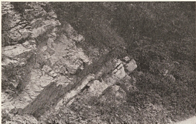
Sl. 22. Skladnat zgornjetriasni dolomit v spodnjem delu golice in nerazločno plastnat dolomit z megalodontidnimi školjkami v njenem zgornjem delu. Po A. Ramovšu
