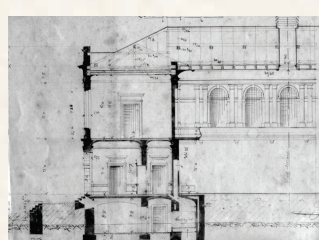
Sokolski dom po načrtu Hraskega leta 1892 Arhiv RS
