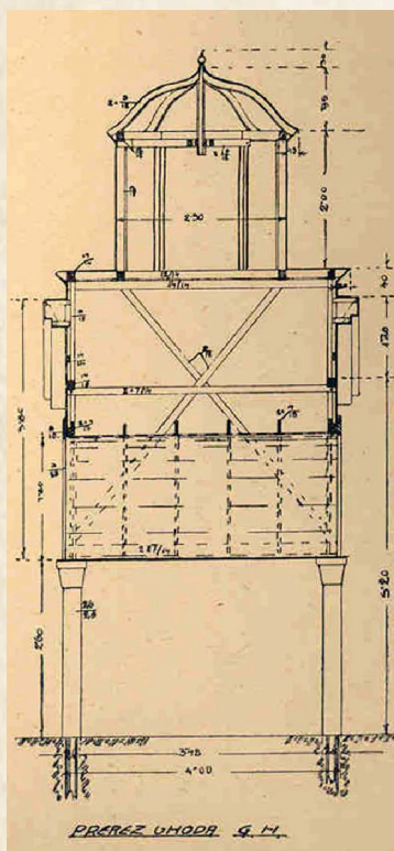
Prerez vhoda Arhiv Fakultete za šport
