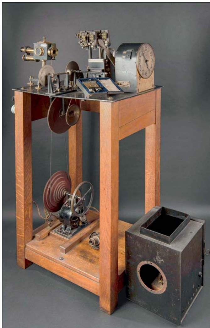
Slika 36: Fonoskop (galvanometrski oscillograf) s katerim je leta 1913 Ivanu Regnu uspelo kot prvemu na svetu grafično prikazati čirikanje poljskega murna ( Gryllus campestris ). Zvočni signal murna, ki je čirikal v kletki, je sprožil iskrenje elektrod, kar je zabeležil premikajoči se filmski trak. Levo je pogonsko kolesje, v sredini registrirni aparat za zapis zvočnih nihajev na filmsko podlago in desno je ura, ki je krmilila delovanje celotne naprave (SITAR 1987).
