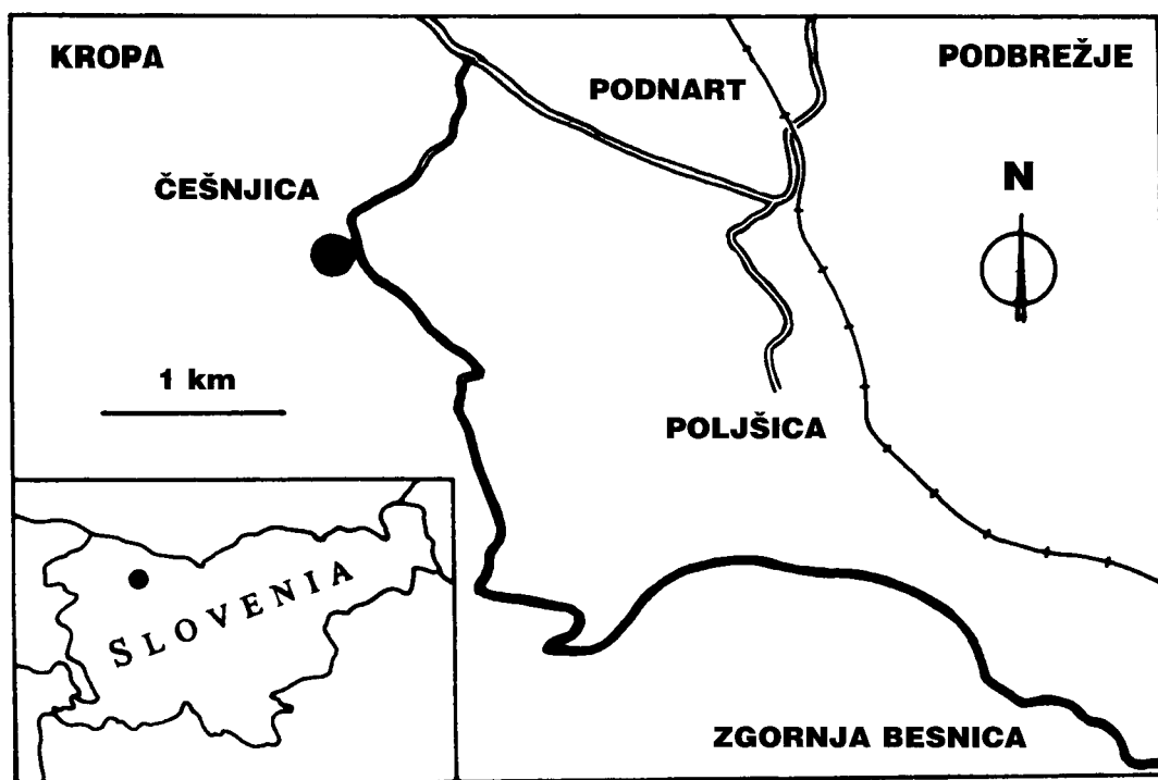
Sl. 1. Položaj nahajališča oligocenskih morskih ježkov pri Češnjici blizu Poljšice Fig. 1. Location sketch map of the Oligocene sea-urchins from Češnjica near Poljšica
