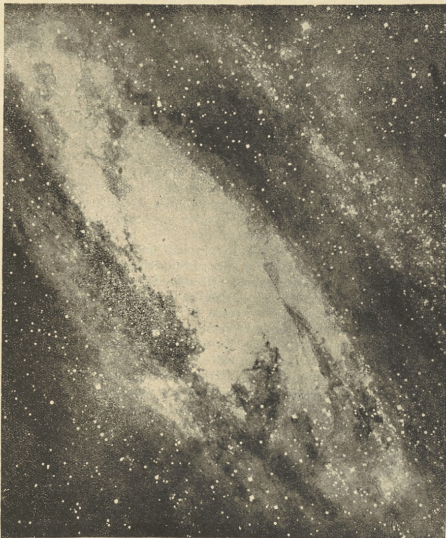
Velika špiralna meglenica, več milijonov svetlobnih let od nas, sestojęča iz mnogo milijard sonc in plinov, iz katerih se bodo zgostile nove zvezde. (Meglenica v Andromedi)
