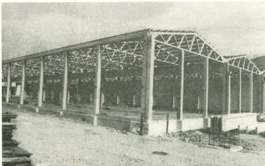
Konstrukcija skrajšane proizvodne hale stoji
