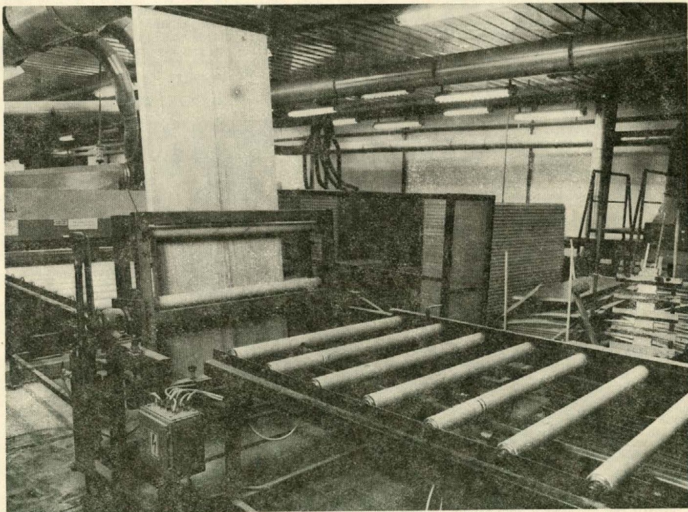
Obračanje vratnih kril na liniji za brazdanje in brušenje vratnih kril v TP Prevalje je sedaj avtomatsko. To je tehnična izboljšava Ivana Kompreja in sočelavcev v vzdrževalni skupini.
