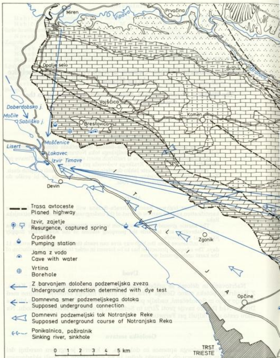
Sl. 1. Hidrogeološka karta Krasa
