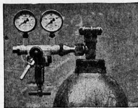
REDUČNI VENTIL »AGA-RUŠE« Z NAVZDOL OBRNENIM REGULIRNIM VJAKOM.
