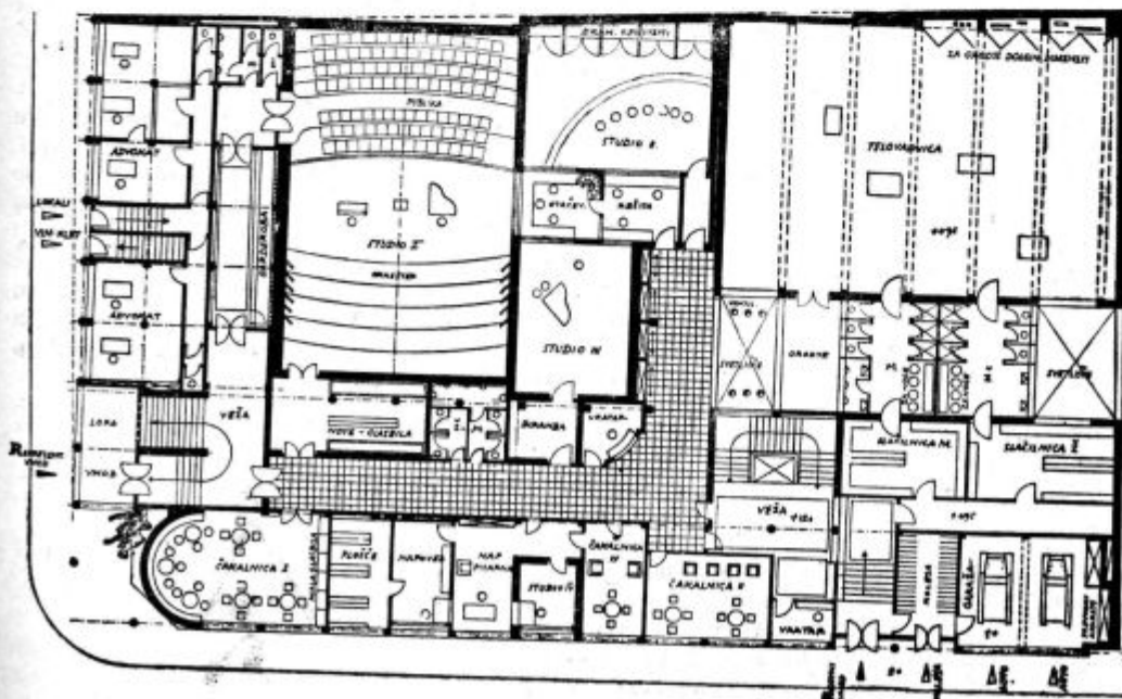
Tloris pritličja »Slov. doma« po osnutku ing. arh. M. Terpina. Daljša stran gleda na Kolodvorsko ul.
