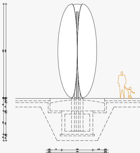
POGLED A - A M 1:50
