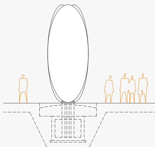
POGLED B - B M 1:50
