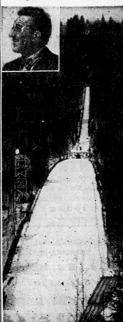
125 metrska skakalnica v Planici, na kateri bodo nedeljski smuški poleti je največja in najboljša na svetu. Levo zgolj njen konstruktor inž. Bloudek
