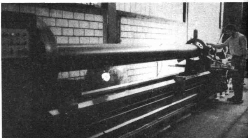
Iz TCP Djuro Salaj: brušenje valjev za papirne stroje je zelo zahtevno opravilo. (Foto: Črt Čargo)
