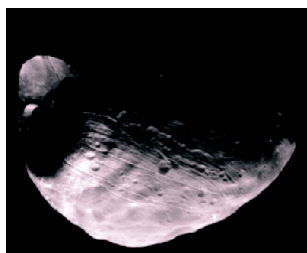
Fobos — Marsu bližja luna
