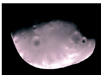
Deimos — druga Marsova luna
