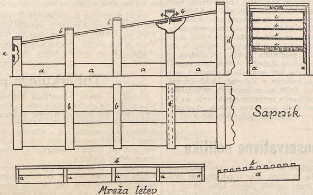
Sapnik: a) stranske odprtine b) pokrovne odprtine c) čelna odprtina d) priključek na žrelo sapnika. Mreža letev: a) podložene deske b) nabite letve.
