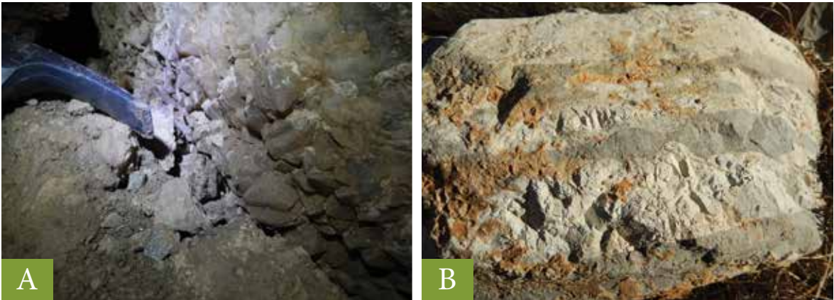
Slika 3: Veliki kristali kalcita v Jelenovem rogu (A) in menjavanje plasti dolomita in klastitov (B) na Čemšeniški planini Foto: Alenka Jelen, januar 2017.
