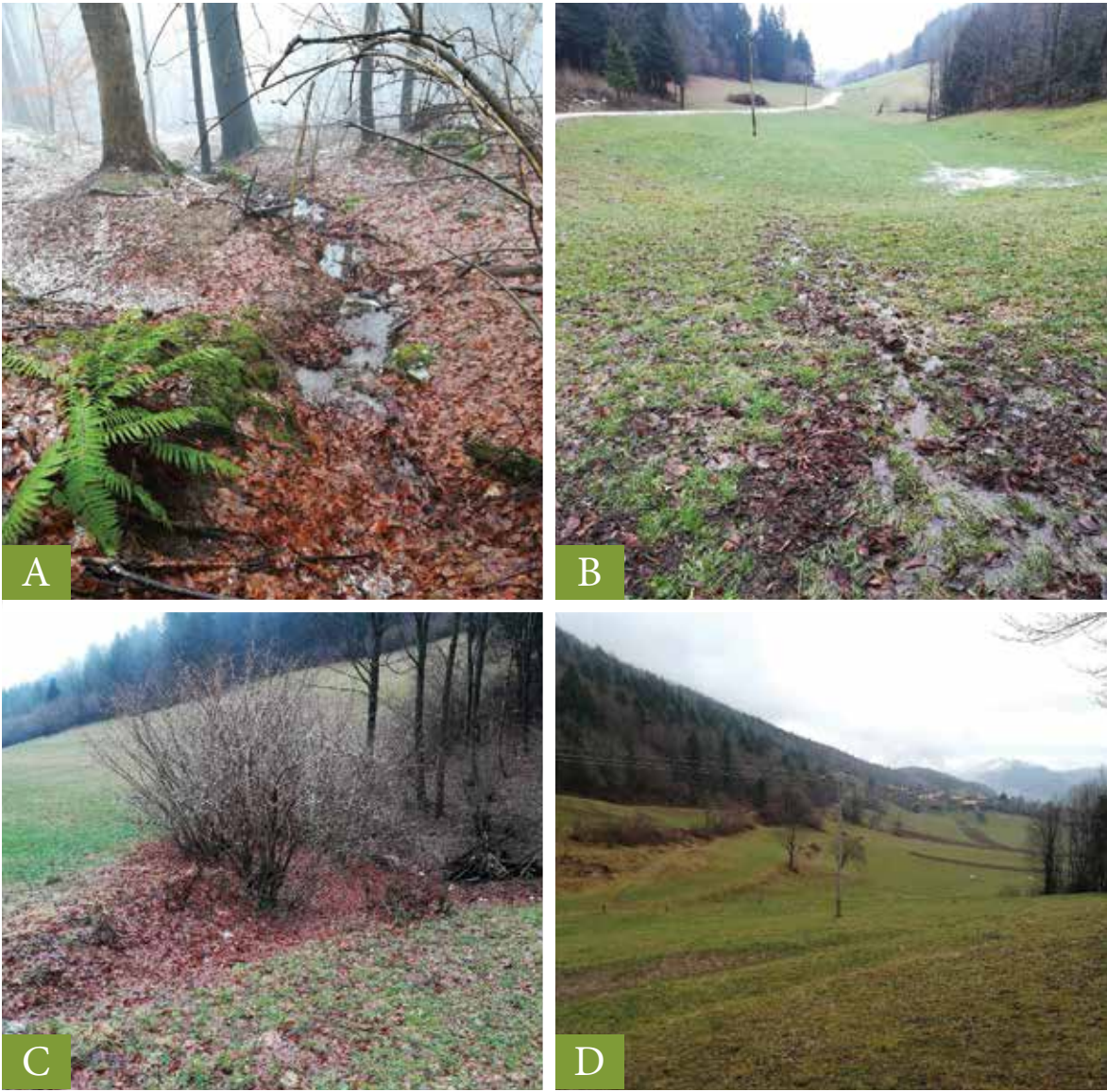
Slika 4: Na območju prelaza Lipa so številni izviri vodotoka (A), ki ponika v slepi dolini nad Vologo (B). V spodnjem delu doline je krajša slepa dolina (C), pod naseljem Vologa pa večja kraška kotanja (D).
