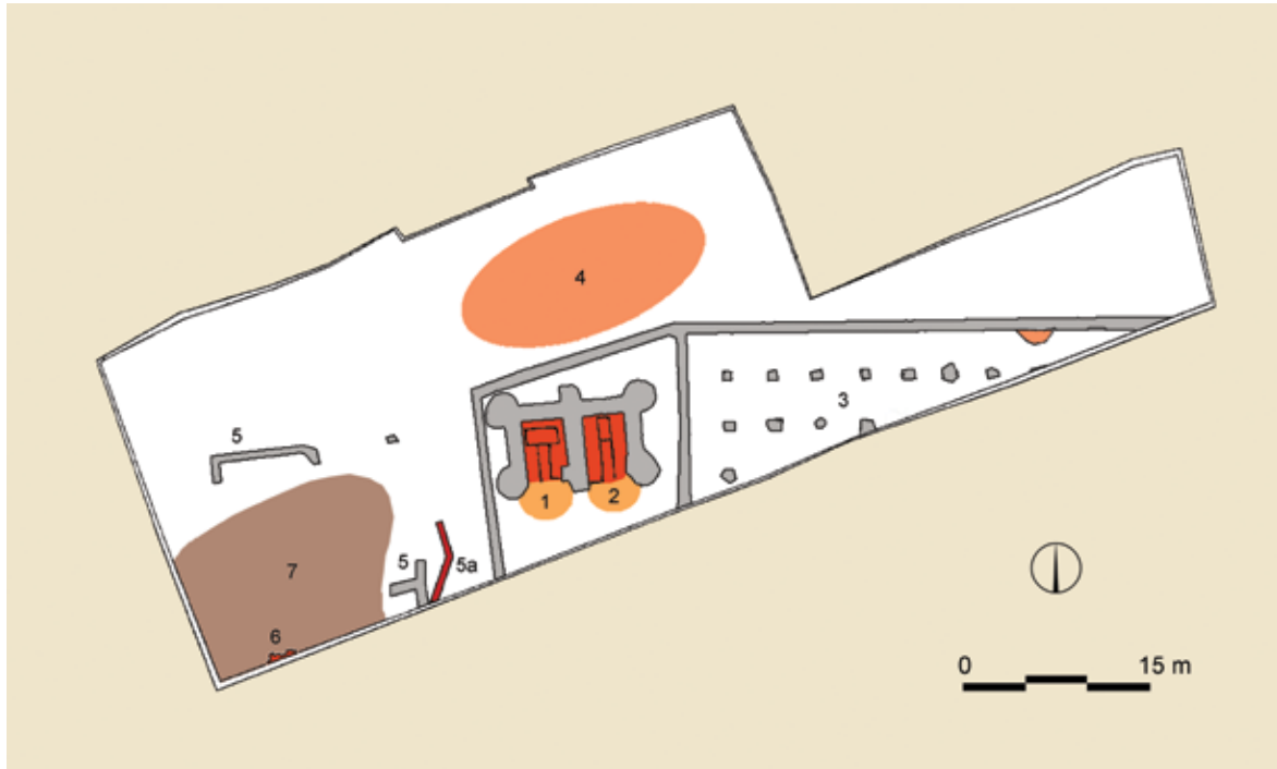
Slika 2: Tloris odkritih arheoloških struktur na najdišču: 1– peč 1, 2 – peč 2, 3 – skladišče, 4 – odpadna jama, 5 – ostanki arhitekture, 5a – kanal iz opek, 6 – ostanki peči, 7 – jama s prodom
