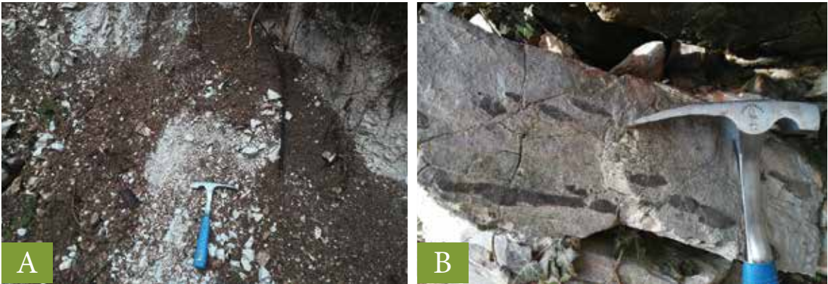
Slika 2: Prevladujoč dolomit (A) in gomolji roženca v apnencu v Merinci (B) Foto: Alenka Jelen, december 2017.
