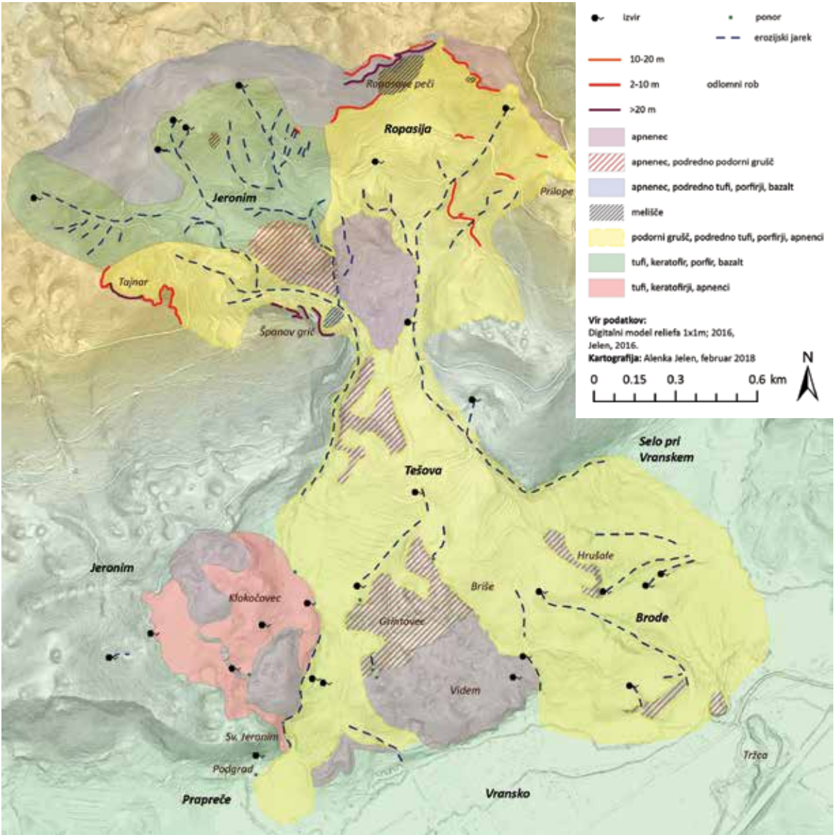
Karta 2: Območje fosilnega plazu nad Vranskim
