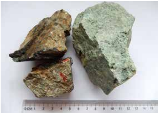
Slika 1: Podorni material – debelo-zrnati zeleni tuf
