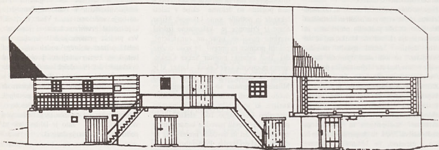
Risba Budnarjeve hiše - južna fasada oz. dvorišna stran (Andrej Kocjan, študent Fakultete za arhitekturo).
