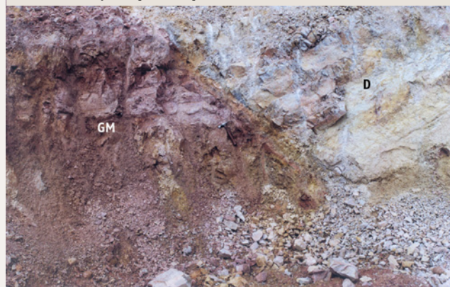
56 Grödenski peščenjak in muljevec (GM) v tektonskem stiku z dolomitom (D).
