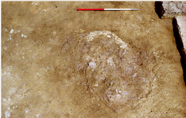
20 Deponija rumenega meljevca in rdečega muljevca, sektor 2.
