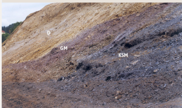
54 Golica pri Višnji Gori. V zaporedju si sledijo: črn karbonski skrilavi muljevec (KSM), rdeč grödenski muljevec in peščenjak (GM) ter dolomit (D).
