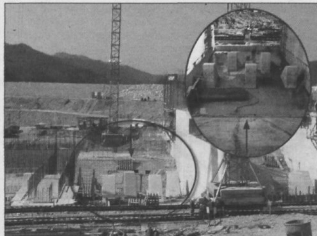
Eno izmed prelivnih polj na HE Blanca v času gradnje. Večji posnetek prikazuje polje v smeri proti toku reke, izrez pa v smeri toka Save. Puščici označujeta smer plovbe kanujev. Foto: arhiv PO
