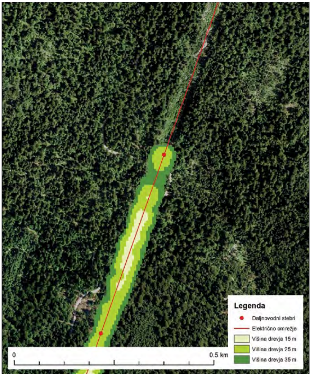
Slika 6: Spreminjanje širine daljnovodne preseke z upoštevanjem različnih višin drevja in reliefa (namenoma je prikazan del, kjer se je naša analiza zaključila, da je viden koridor enotne širine)
