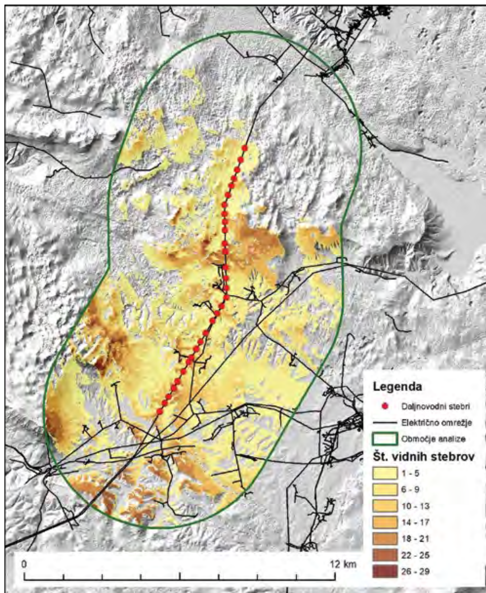
Slika 4: Vidnost daljnovodnih stebrov
