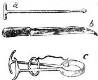
Pod. 27. Orodje za lov voluharja. a tipalo, b trebilo, c klešče (past) za voluharja.
