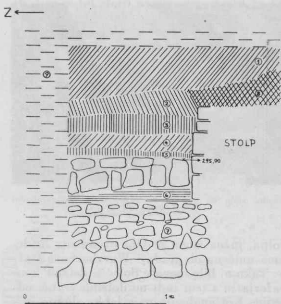
Profil I.
