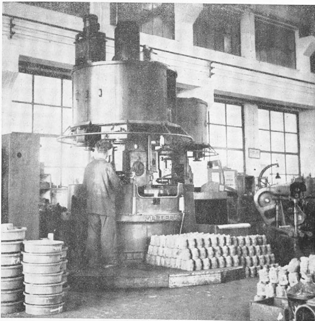
Izdelava kolesnih stavkov. Stroj, ki se mu rad odkriješ, kajti šest funkcij opravlja istočasno in avtomatsko. Tu človek res samo še na gumb pritisne, nastavlja surove in odvzema obdelane kose.
