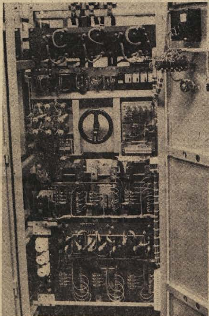
Pogled v notranjost silicijeve usmerniške naprave za napajanje avtomatskih telefonskih central (Foto: M. Jakopec)
