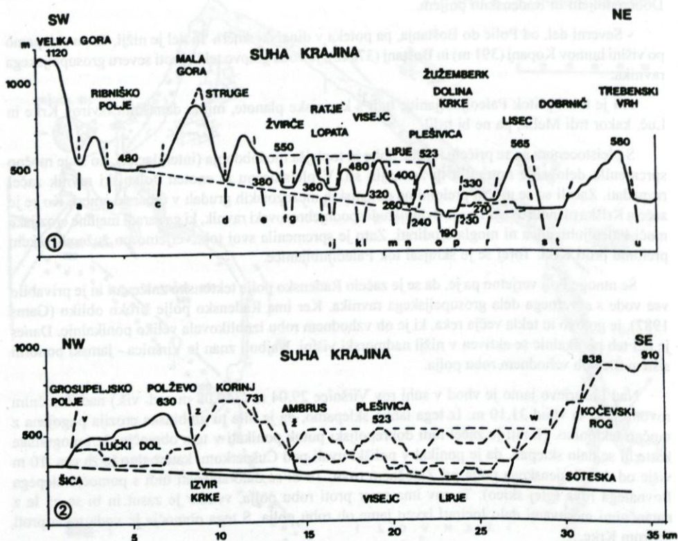
Sl. 2. Prečni (1) in vzdolžni (2) morfološki presek zahodne Suhe krajine, a-u reliefne strukturnice na prelomnih conah, rebri: a - velikogorska, b - bukovniška, c - malogorska, d - dobrepoljsko-kukovska, e - seška, f - žlebenska, g - zvirška, h - retlanska, i - jarška, j - lopaška, k - selska, l - visejska, m - cerska, n - gradenska, o - stranska, p - žužemberška, r - zališka, s - dobrniška, t - vrbovska, u - trebenjska, v - slivniška, kriška, z - znojilsko-kočevska, ž - ambruška, w - smuška.
