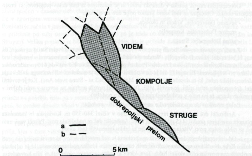
H a b i č. P., 1988, Tektonska pogojenost kraškega reliefa zahodne Suhe Krajine
