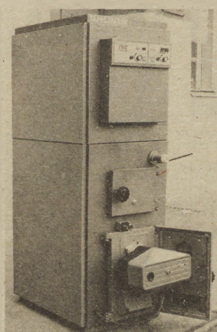
MODEL UL — Univerzalni toplovodni kotel z ali brez boilerja za ogrevanje sanitarne vode. Možnost uporabe tekočih, plinastih in trdih goriv.
