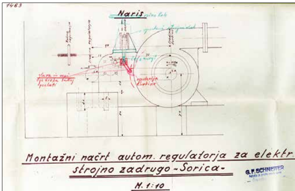
Načrt za montažo avtomatskega regulatorja podjetja G. F. Schneider iz Škofje Loke, poleti 1939.
