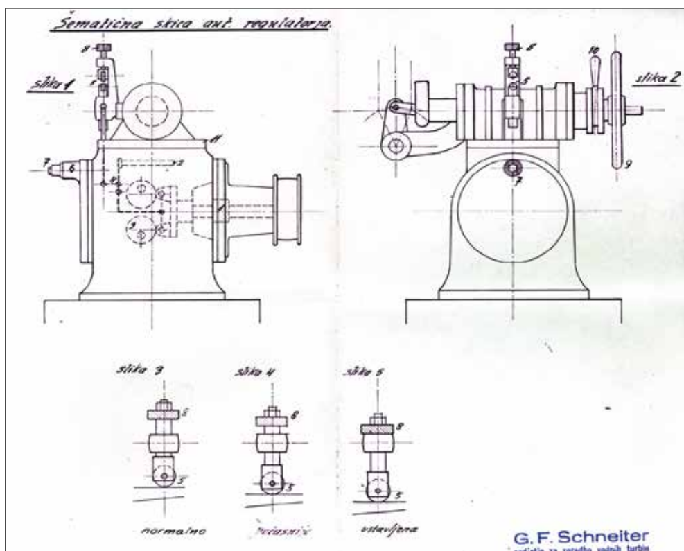
Shematična skica avtomatskega regulatorja podjetja G. F. Schneider.
