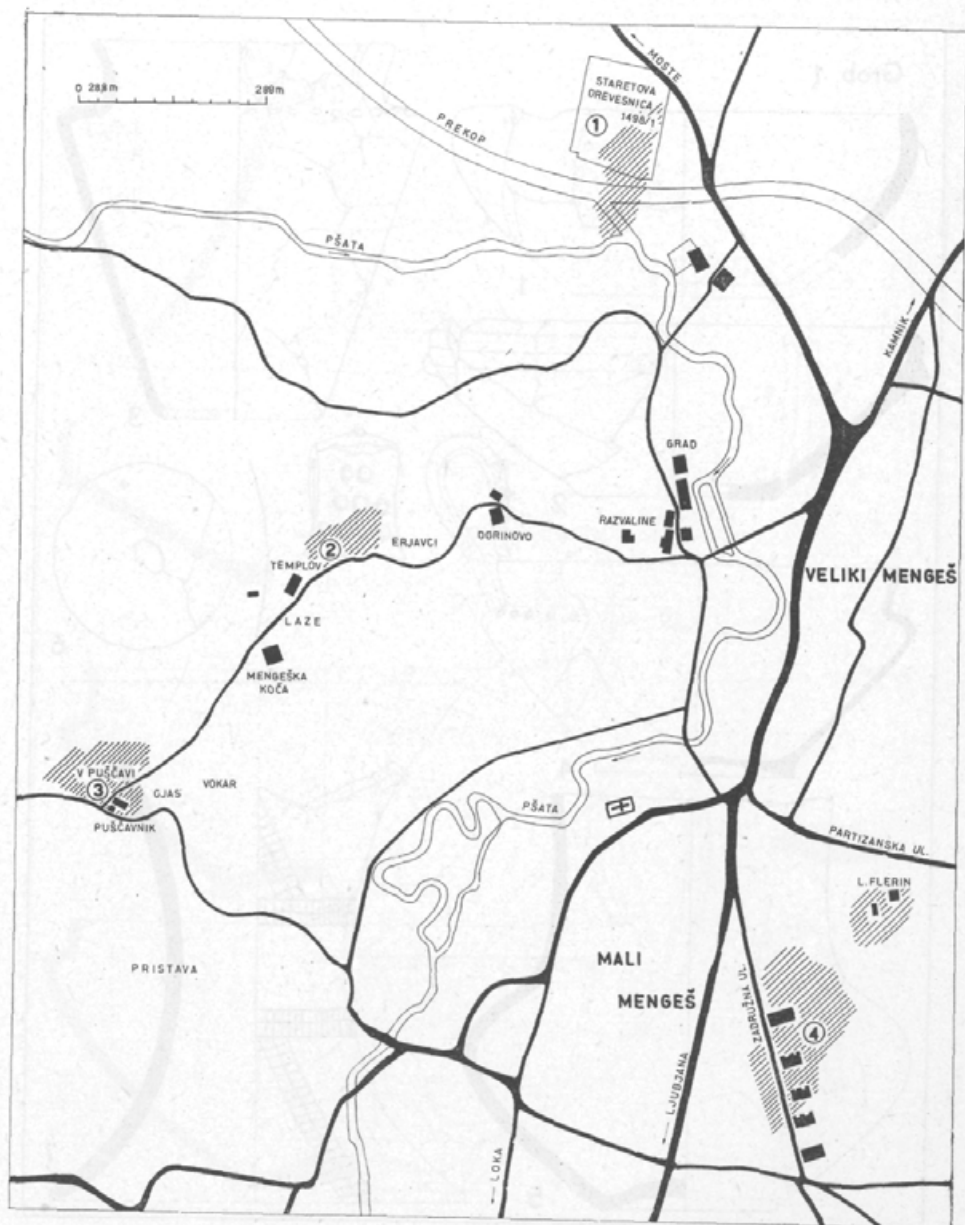
Karta 1 — Arheološka najdišča v Mengšu
