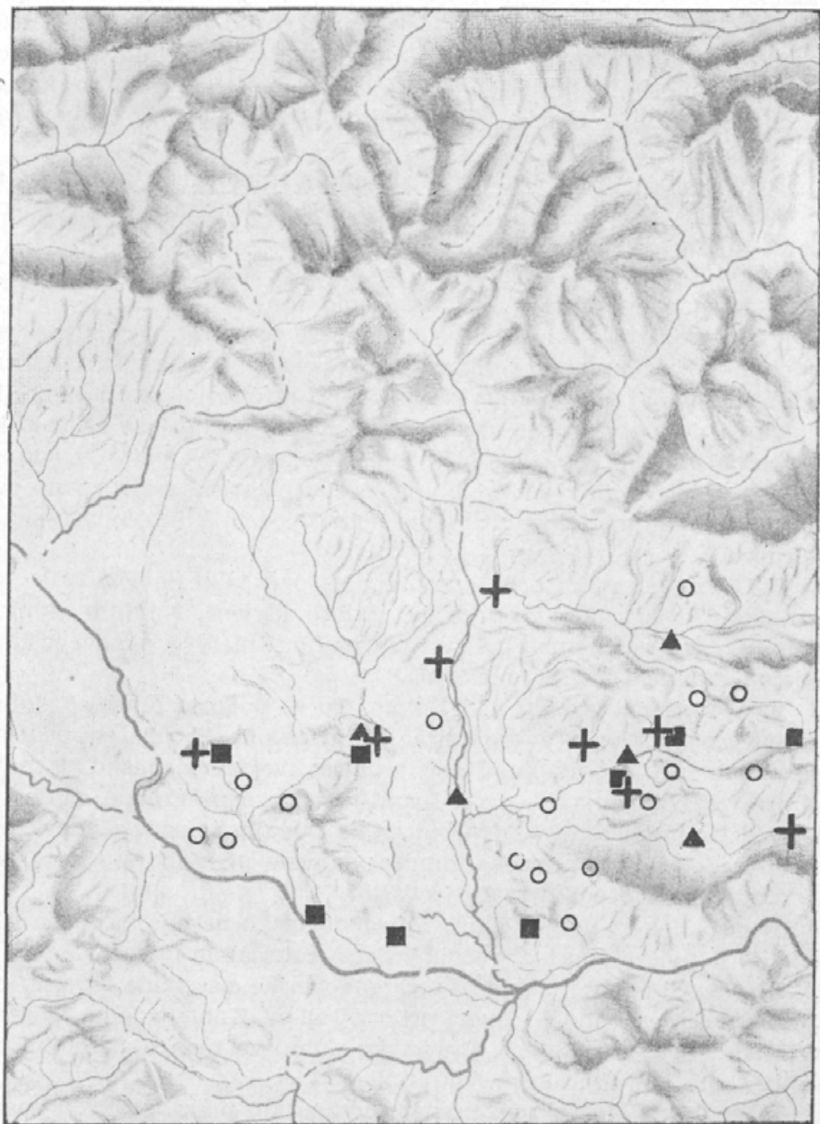
Halštatska in latenska najdišča kamniškega področja
