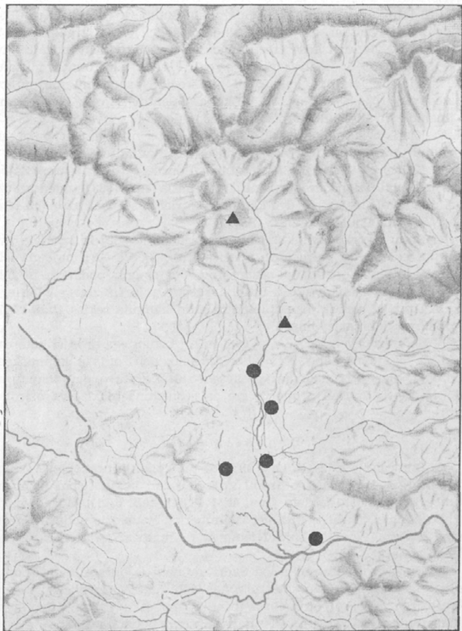
Paleolitska (Δ) in neolitska (●) najdišča kamniškega področja
