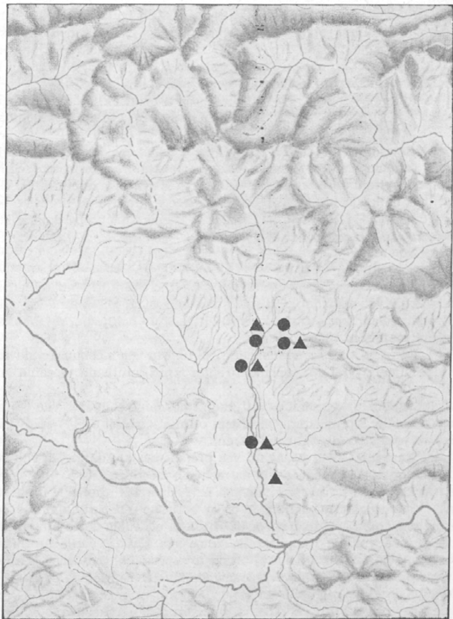
Bronastodobna ( \triangle ) in žarnogrobišna ( \bullet ) najdišča kamniškega področja
