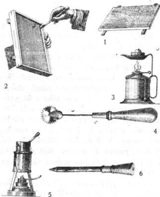
Deščica za utiranje žice. — Pritrjevanje satnic z voskom. — Svetilka za pritrdjevanje satnic. — Kolesce za utiranje žice. — Mali topilnik za vosek. — Cevka za zalivanje satnic pri gornjem robu.
