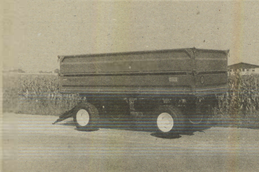
Traktorska prikolica tip »TEHNOSTROJ DDK 500«
