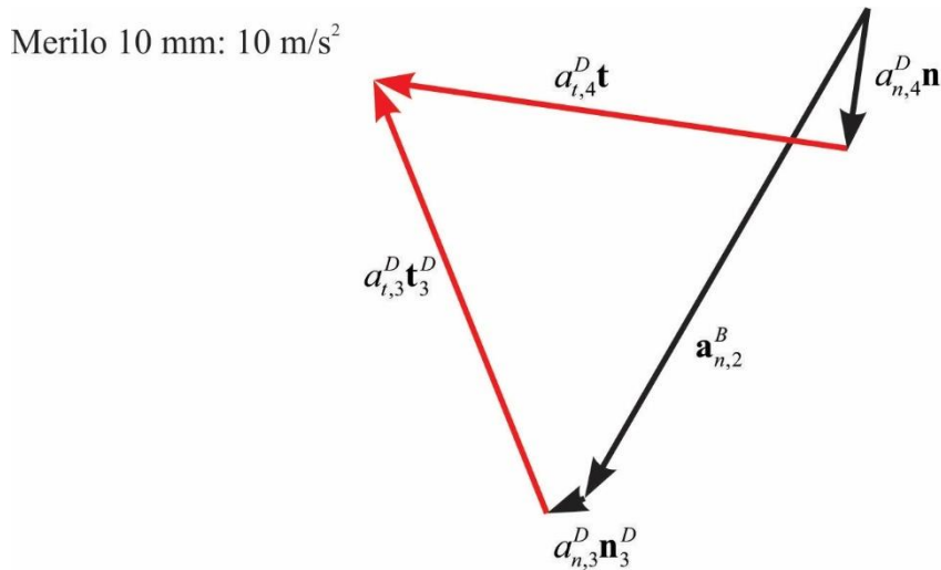
Slika 10. Poligon pospeškov za točko D.
