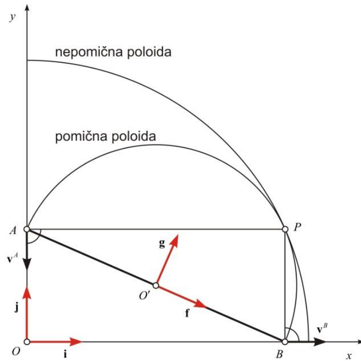
Slika 23. Gibanje palice – kotaljenje poloida.
