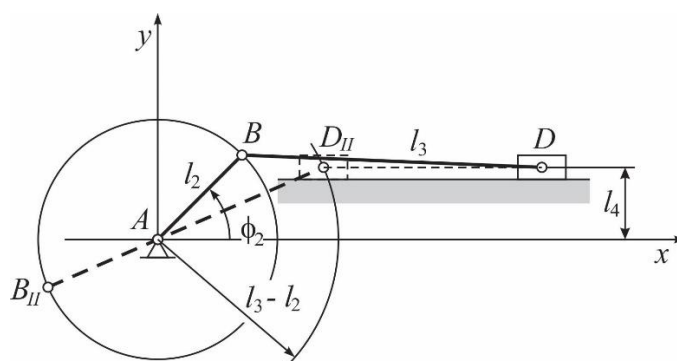
Slika 83. Ročični mehanizem.
