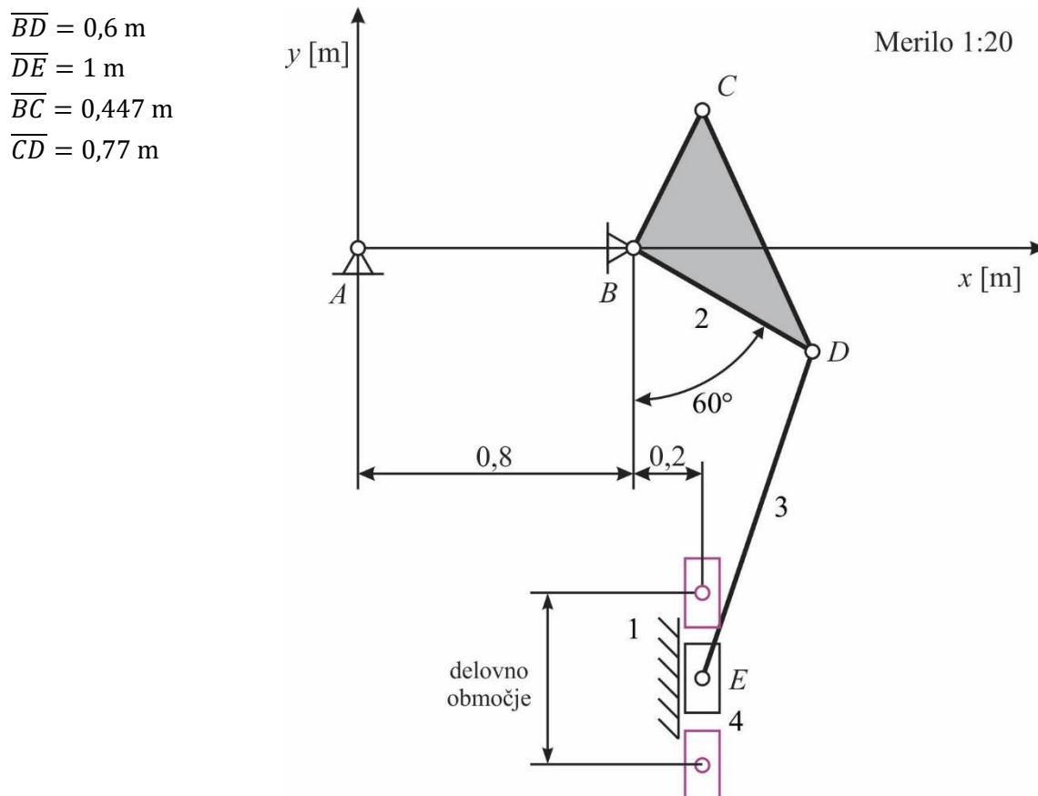
Slika 20. Delovno območje ročičnega mehanizma z drsnikom, brez pogonskega podsistema.
